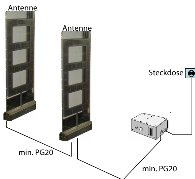
Verkabelungsschema Einzelgate
